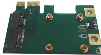
F-ADP-MINI-PCIE
